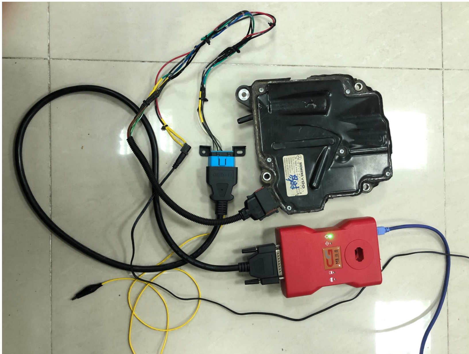
实物接线图
